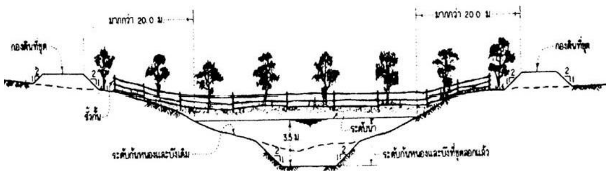
ลักษณะและรูปแบบทั่วไปของการขุดลอกหนองน้ำและบึงธรรมชาติขนาดเล็ก
