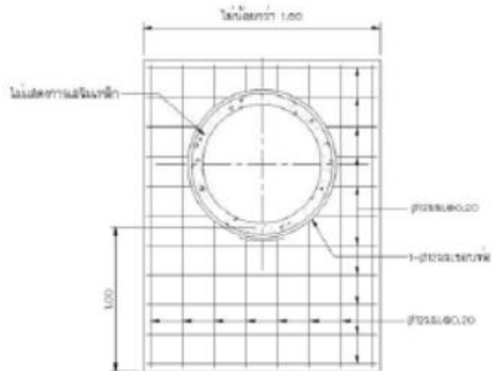
ขยายการเล็งเหล็กกำแพงปากท่อและท้ายท่อ
