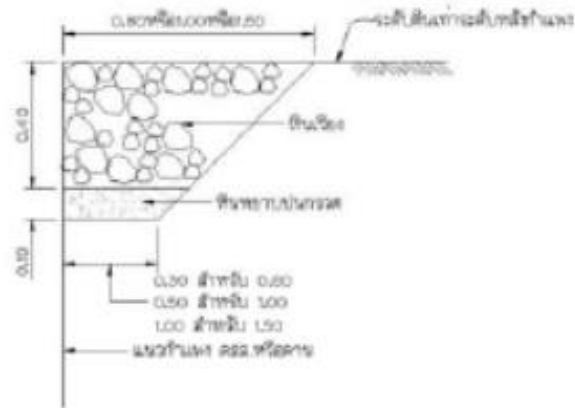
ขยายดินเรียง ② สำหรับกว้าง 0.80, 1.00 และ 1.50 ม. มาตราส่วน 1:20
