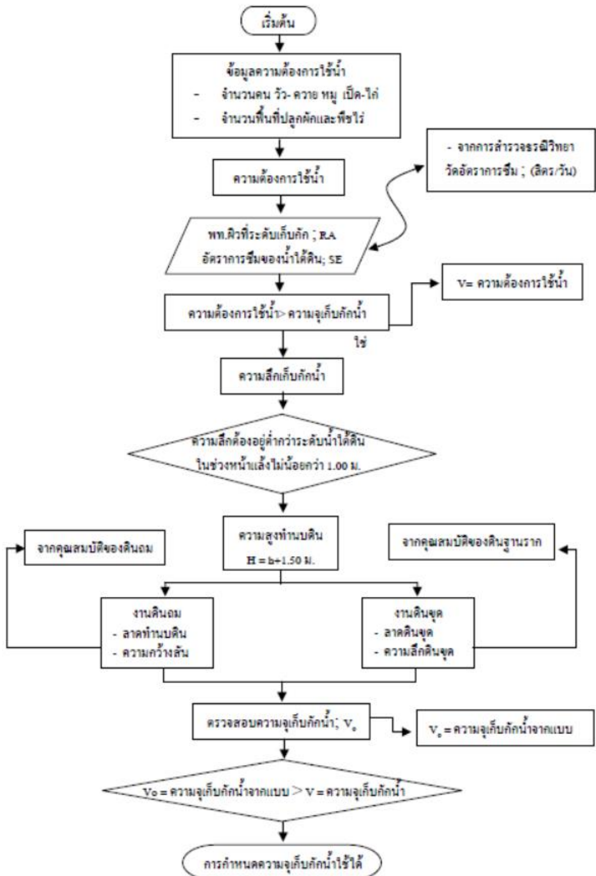
รูปที่ 5.4 แผนภูมิแสดงขั้นตอนการออกแบบสระเก็บน้ำได้ดิน
