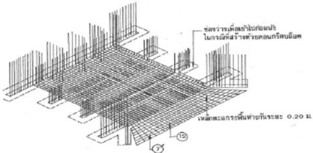
แบบแสดงการวางเหล็กพื้น
