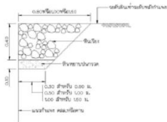
ขยายหินเรียง ② สำหรับกว้าง 0.80, 1.00 และ 1.50 ม.
