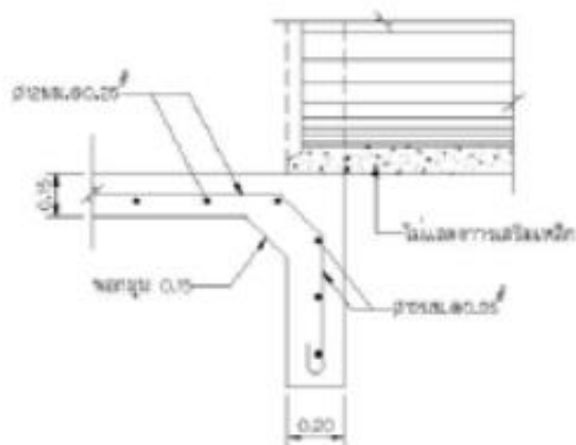
รูปขยาย ③
