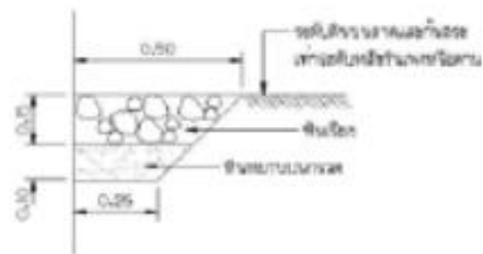
ขยายหินโกลน ① สี่เหลี่ยมกว้าง 0.50 ม.
