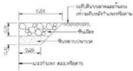
ขยายหินเรียง ① สำหรับกว้าง 0.50 ม.
