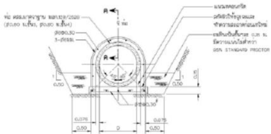
รูปตัดการวางท่อ คลล.
