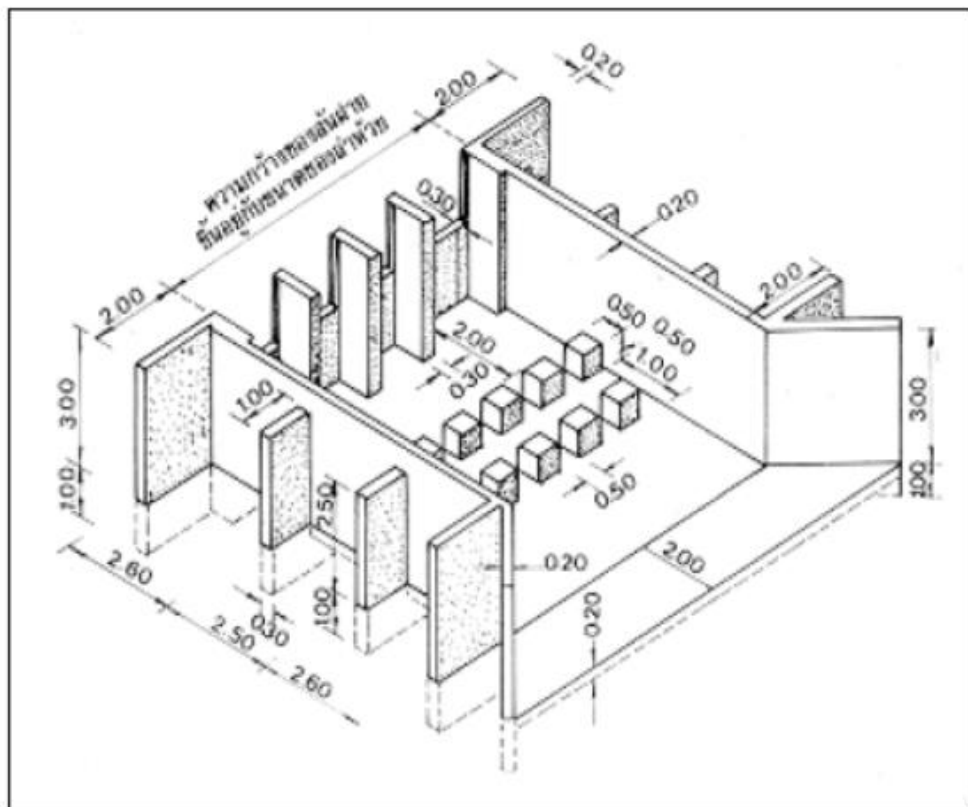
รูปที่ 5.11 แบบมาตรฐานฝ่าย มข.2527 ที่มีส้นฝ่ายสูง 1.50 เมตร หน้าข้างสูง 3.00 เมตร
