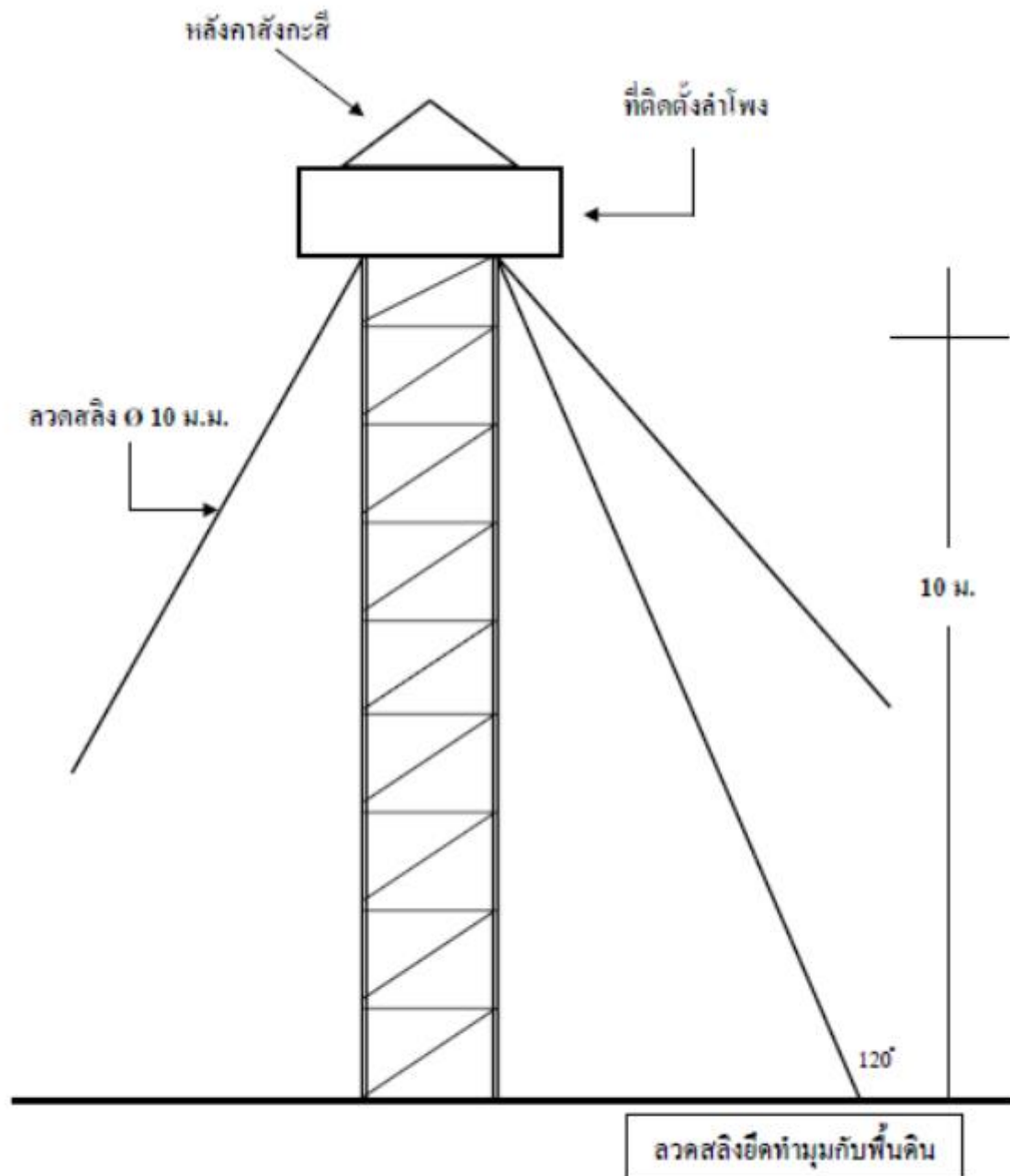
ภาพที่ 2.2 ก ตัวอย่างการใช้ลวดสลิงยึดโครงสร้างติดตั้งลำโพง
